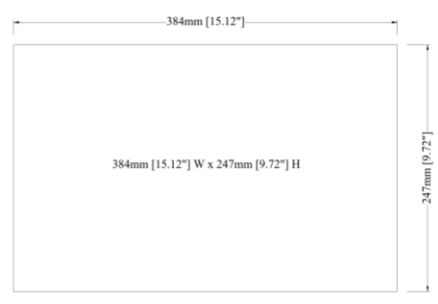
Cutout Dimensions
