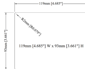
Cutout Dimensions
