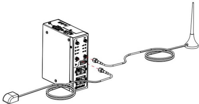
GPS Antenna
