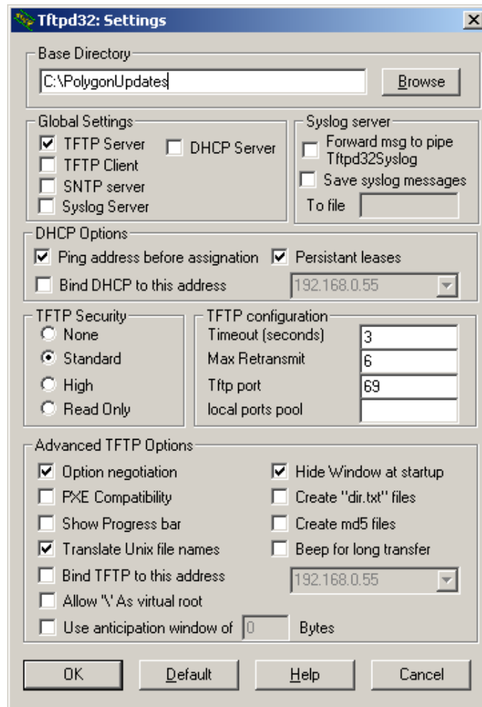
Рис. 17 – Настройки tftpd32
