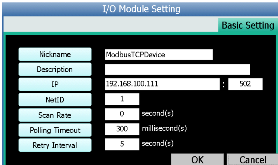
Figure4-38: Modbus TCP I/O module Setting page
