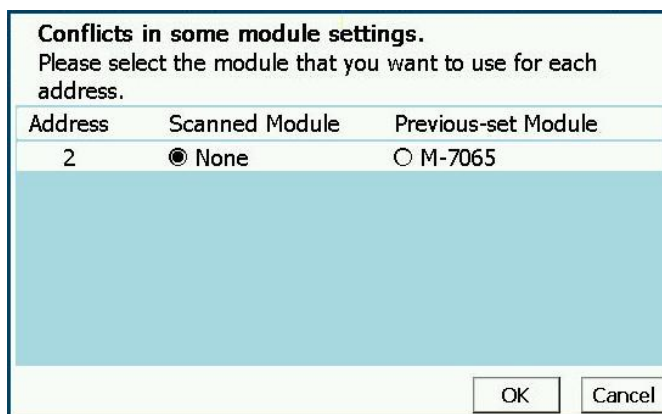
Figure4-32: Select the actual M-7000 module connected to PMD-2201
