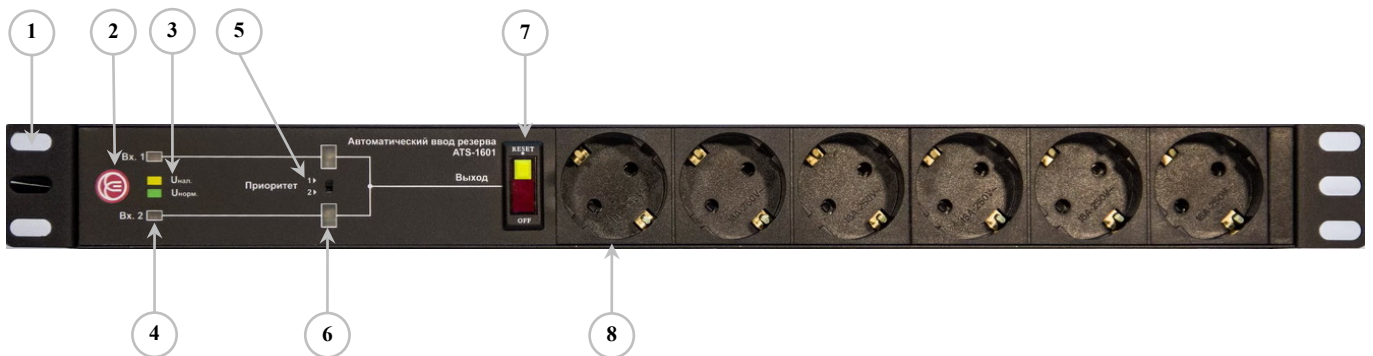
Рисунок 1 – Электронно-механический АВР ATS-1601(P), передняя панель:
