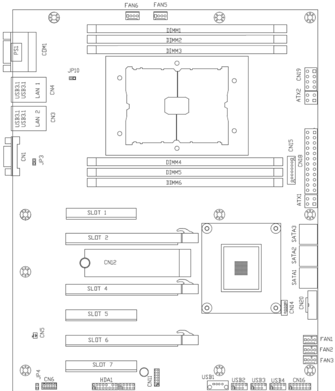
Top side
