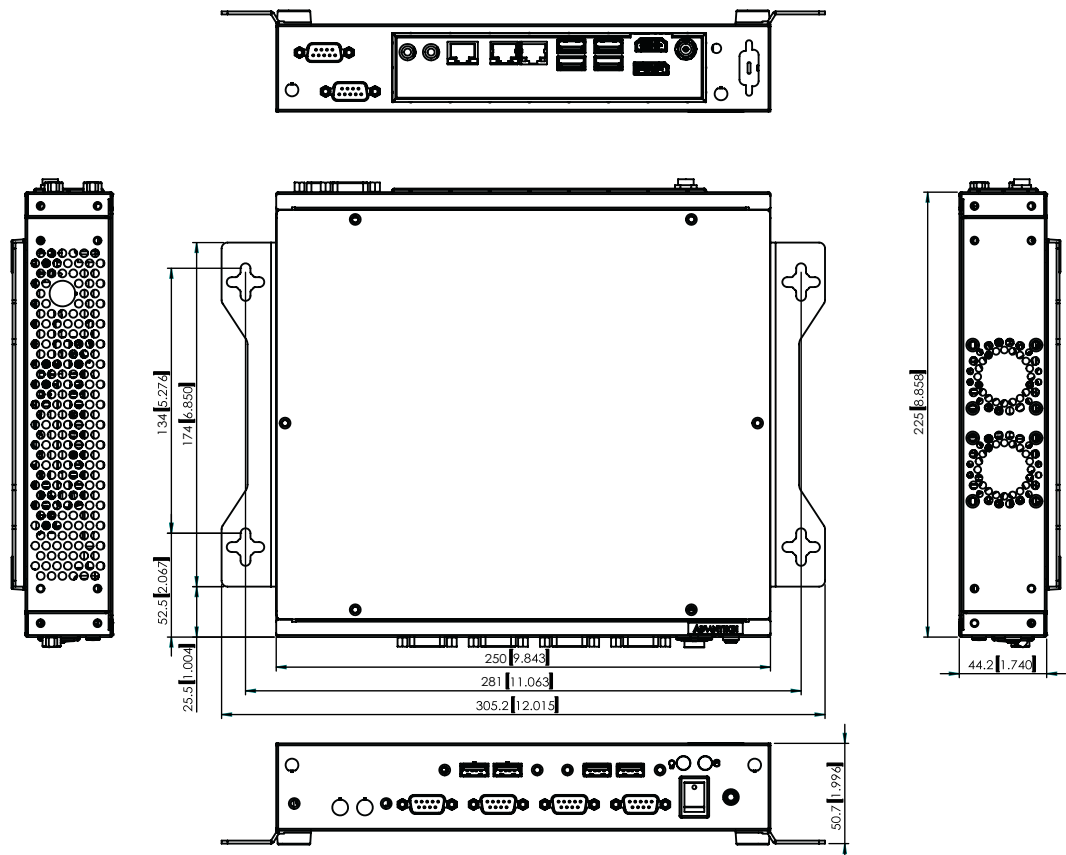
Figure 1.1 Dimensions/ 产品尺寸 / 產品尺寸
