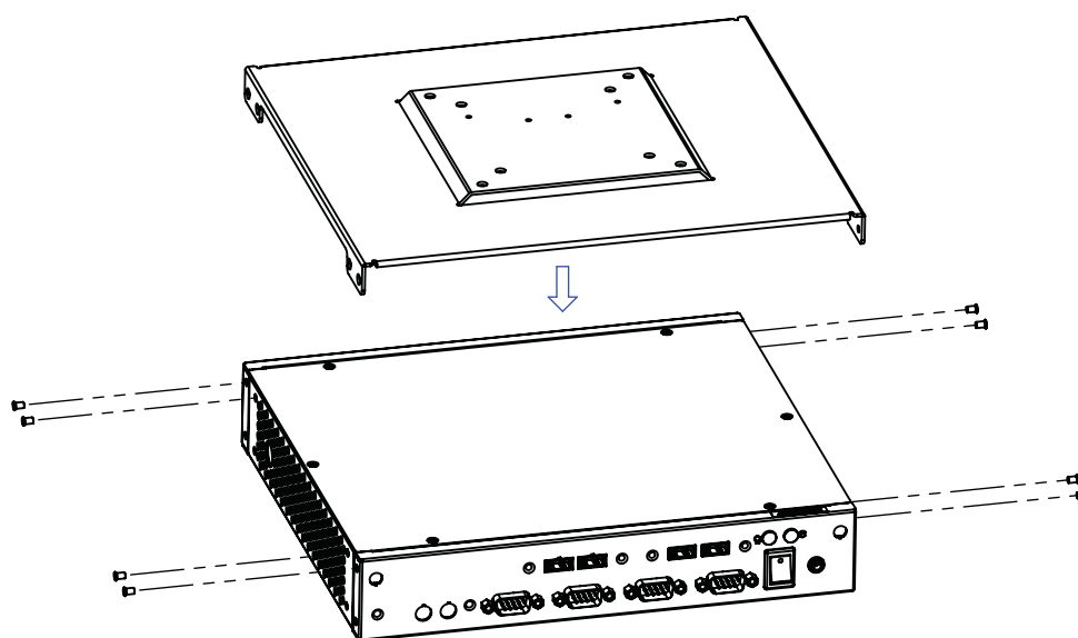
Figure B.2 Installing the VESA Mounting Brackets / 安装机箱底座 VESA 安装架 / 安装机箱底座 VESA 安装架
