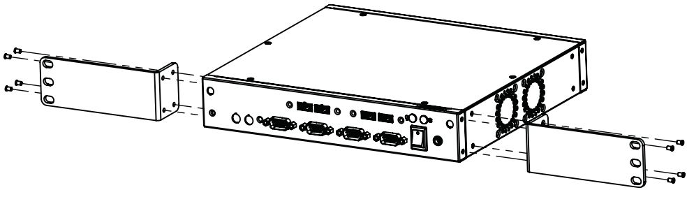
Figure B.3 Installing the Rack Mounting Bracket / 安装机箱 Rack 导轨安装支架 / 安装机箱 Rack 导轨安装支架
