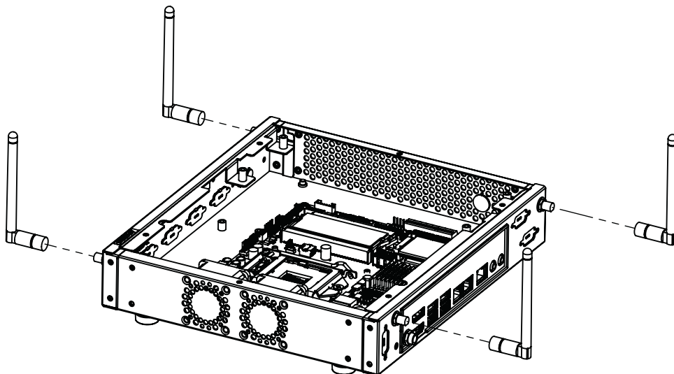
Figure 2.4 Installing the other device/ 安裝其余设备 / 安裝其餘設備
