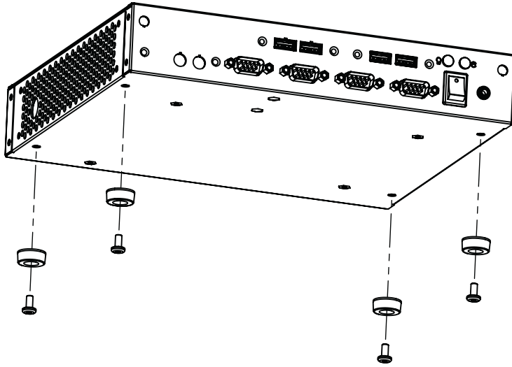
Figure 2.7 Installing Rubber Foot on Bottom Side/ 安装机箱底部橡胶脚垫 / 安裝機箱底部橡膠腳墊
