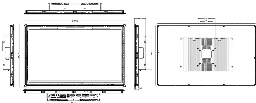
P2381Y-C6 Dimension
