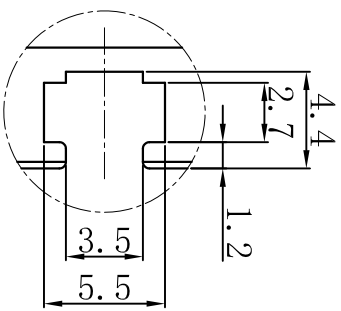
局部A 比例3:1 M3螺母凹槽，安装用
