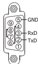
COM2: RS-232
