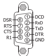
COM5: RS-232
