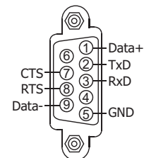
COM4: RS-232/RS-485
