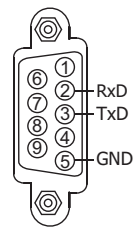
COM1: RS-232
