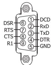
COM5: RS-232
