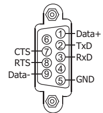
COM4: RS-232/RS-485
