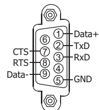
COM4: RS-232/RS-485
