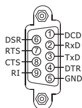
COM1: RS-232
