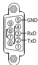
COM2: RS-232
