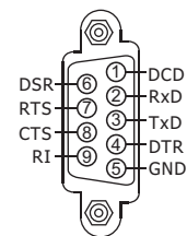
COM3: RS-232
