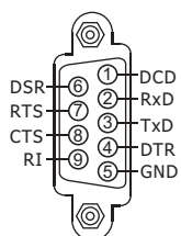
COM3: RS-232
