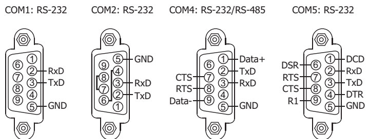
XP-8041-Atom-CE6 COM Port
